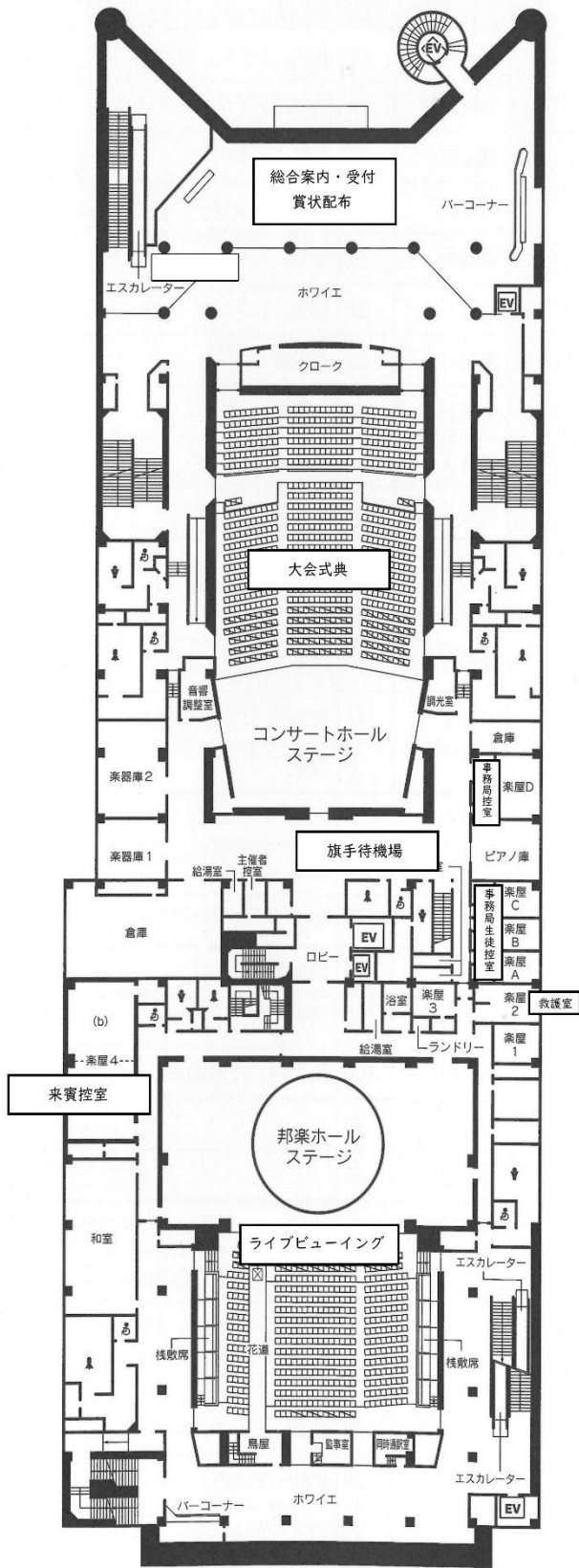
● 2階平面図
