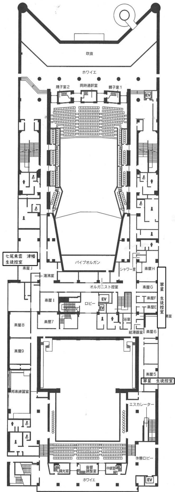
● 3階平面図
